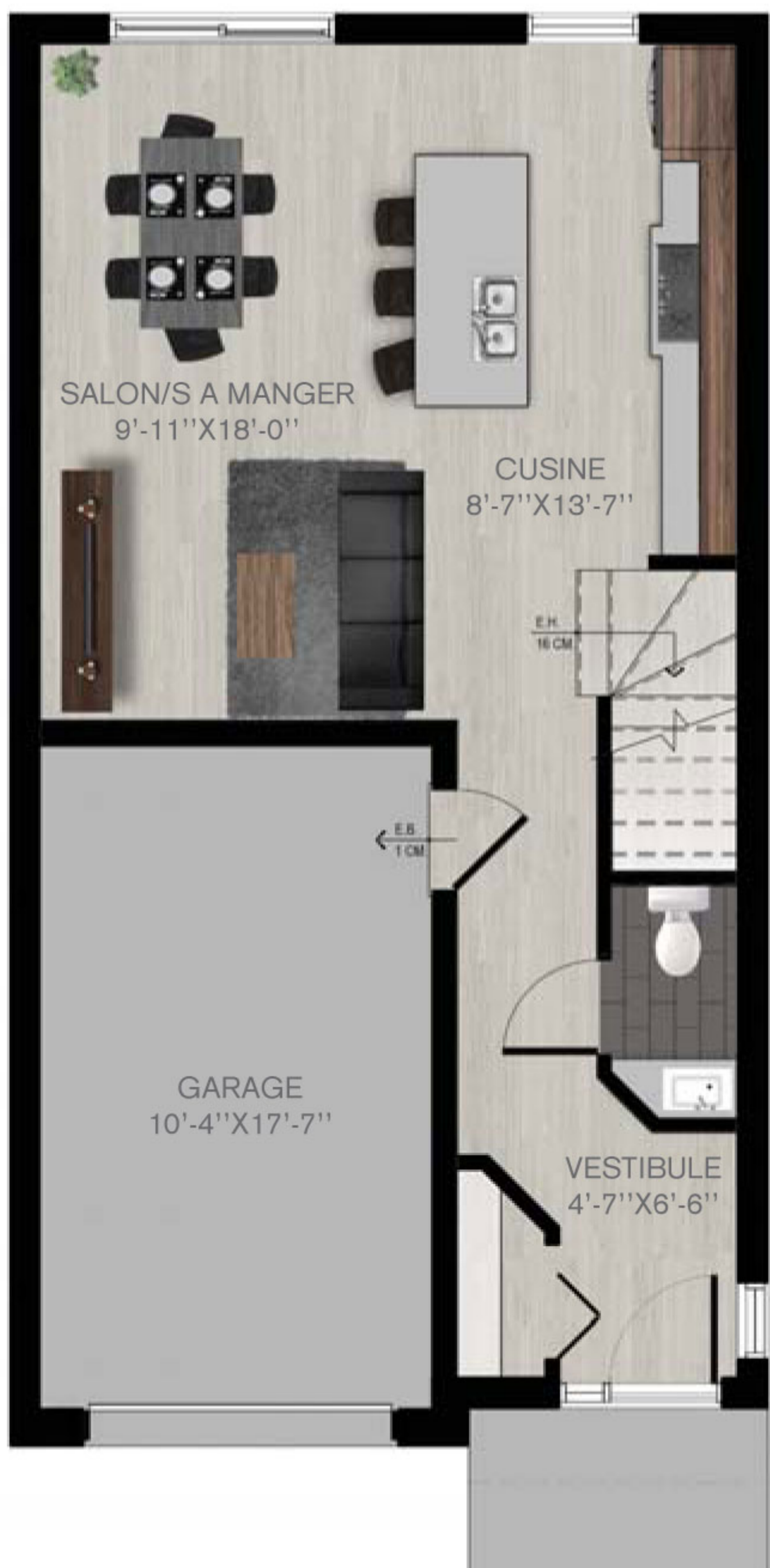
REZ-DE-CHAUSSÉE ± 662 pi 2 NETTE HABITABLE
